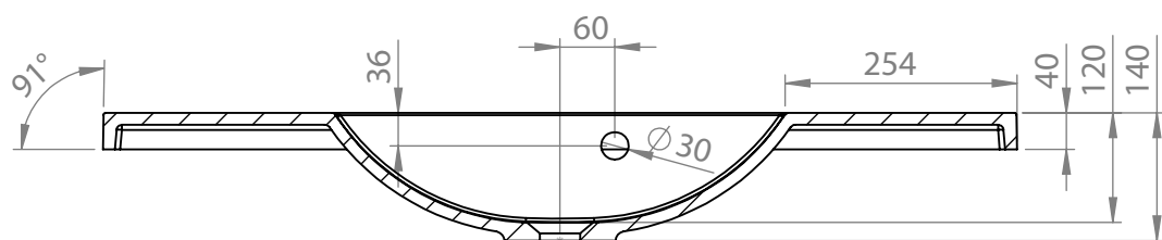
PRZEKRÓJ N-N SKALA 1:9
